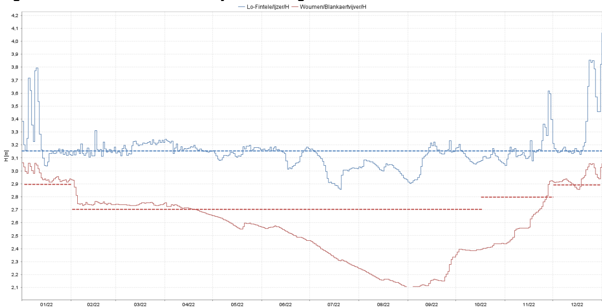
Figuur 5: Waterpeil IJzer en Blankaartvijver t.o.v. streefpeilen 2022
