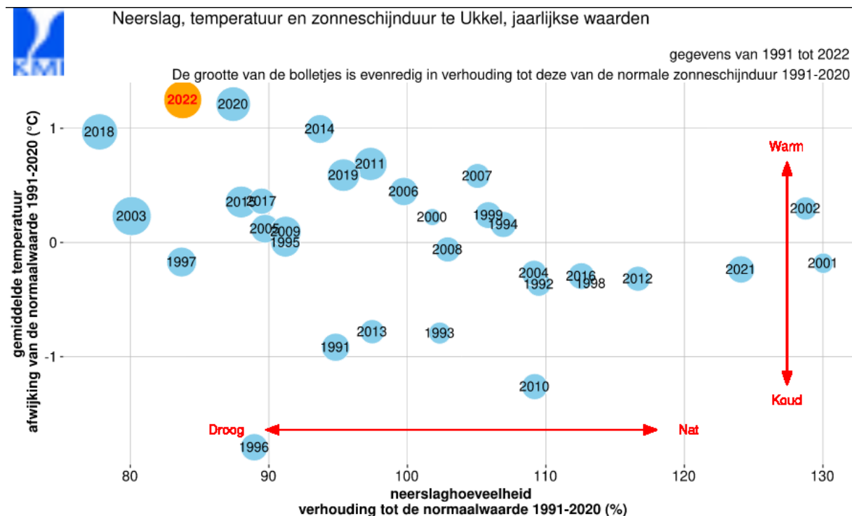
Figuur 1: Neerslag en temperatuur in verhouding tot de normaalwaarde
